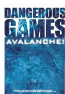
Avalanche!
